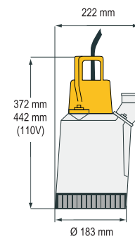
Wymiary (mm)
